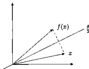
A \notin SO(2, \mathbb{R})
